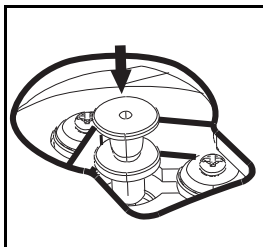
große Öffnung im Plattenteller mit Antriebsrolle - Antriebsriemen montiert
