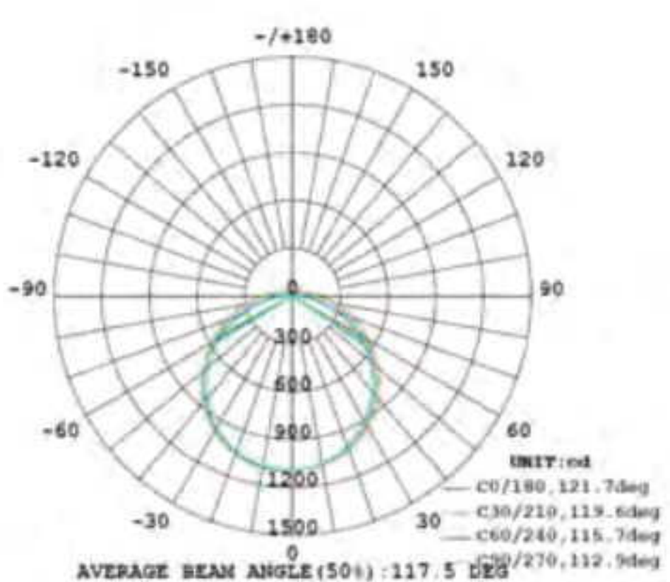
Blaupunkt Linear IP65 36W
