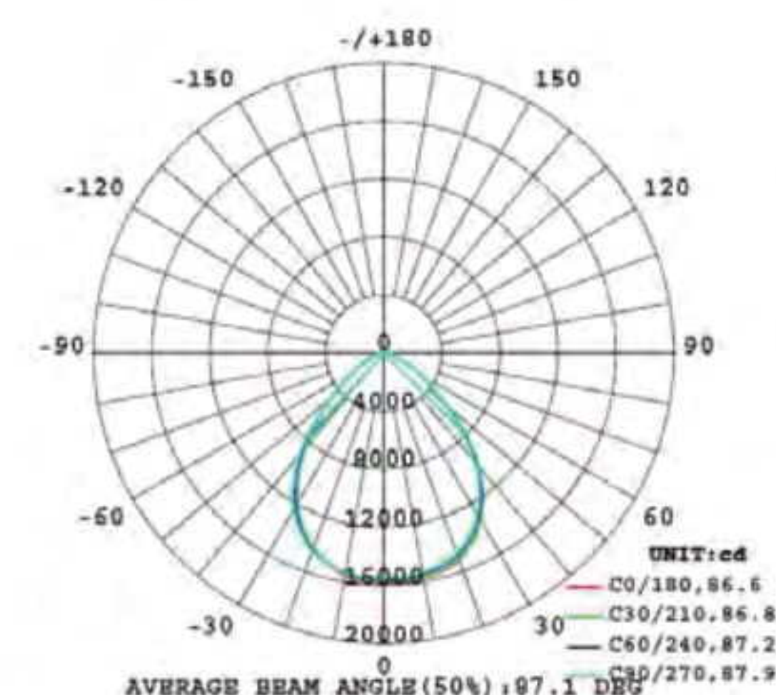
Blaupunkt Highbay Jupiter 200W
