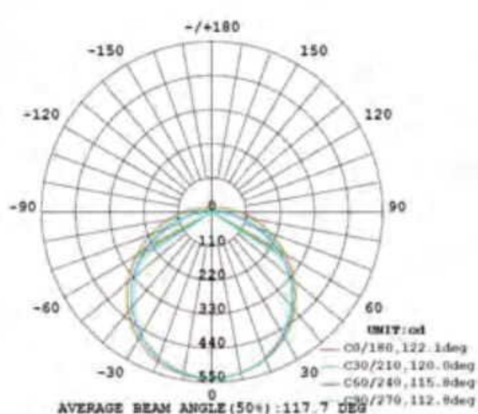
Blaupunkt Linear IP65 18W
