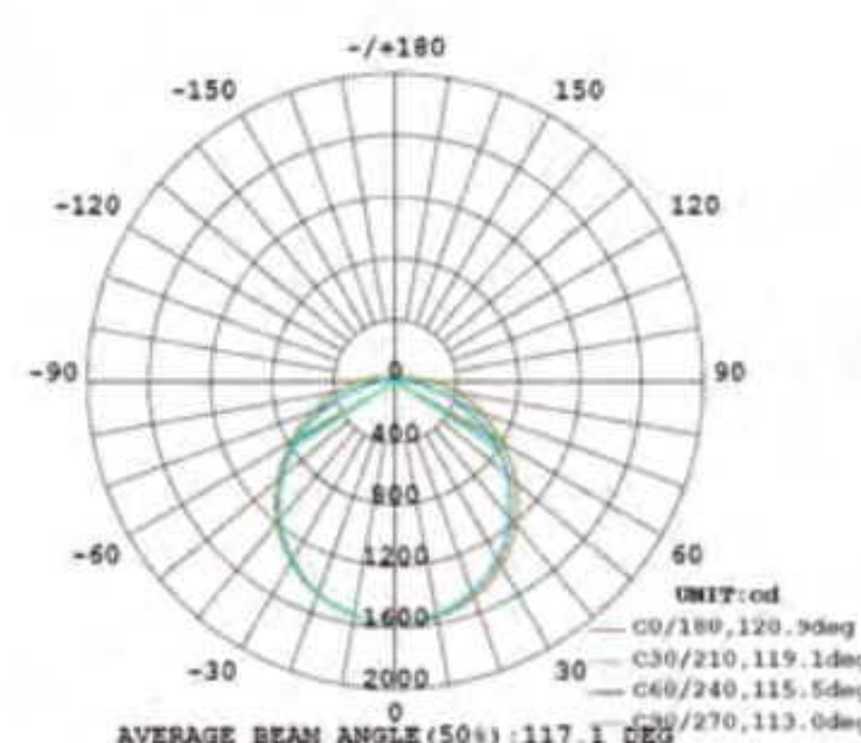
Blaupunkt Linear IP65 50W
