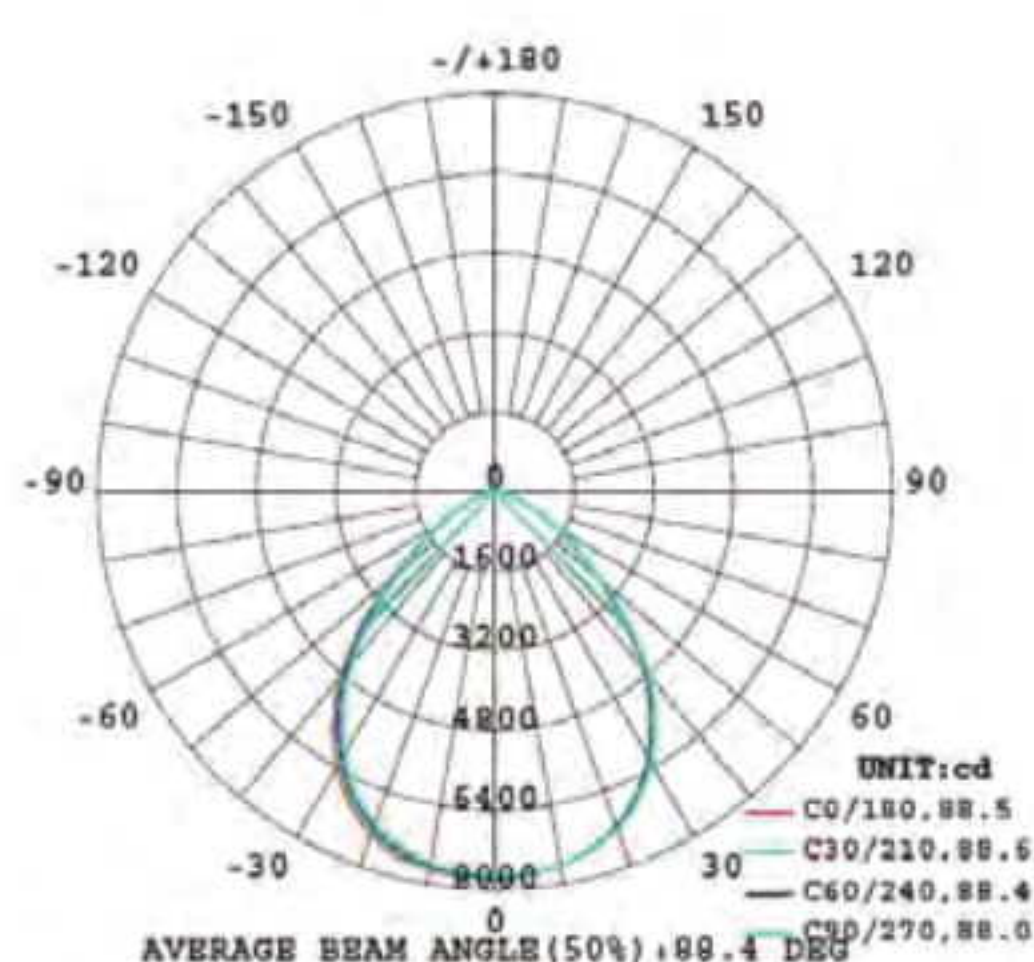
Blaupunkt Highbay Jupiter 100W
