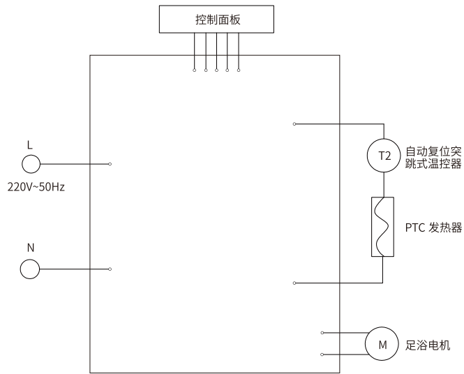
产品电路图
