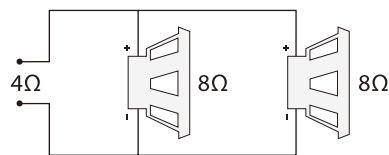
Câblage parallèle
