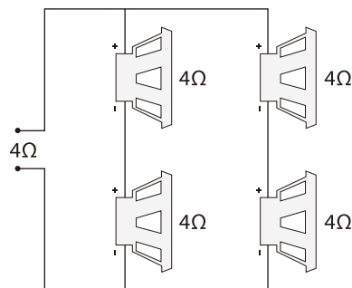
Câblage série/parallèle
