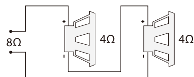
Câblage en série
