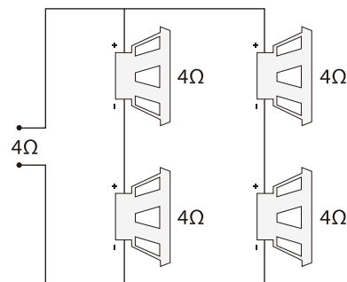
Câblage série/parallèle
