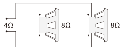
Câblage parallèle
