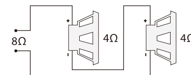
Cableado en serie
